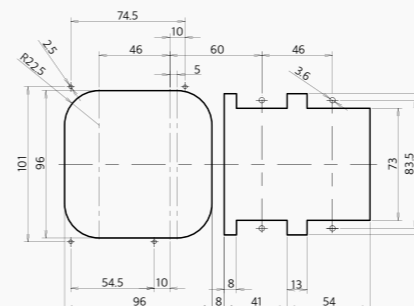
4V-A,B,F형 타공도
