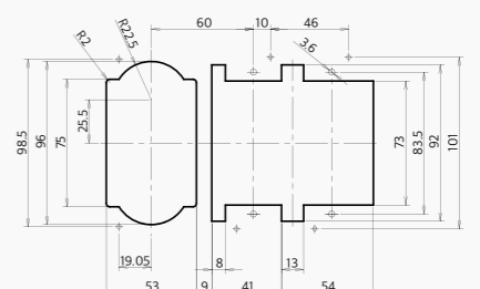
3V-A,B형 타공도
