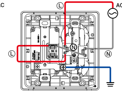
3구용(대기1구+상시2구)
