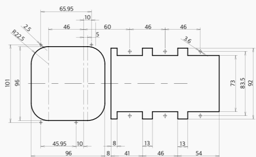
5V-A,F,J형 타공도
