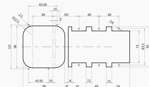
5V-A,F,J형 타공도
