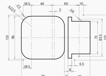
3V-C,E,F형 타공도
